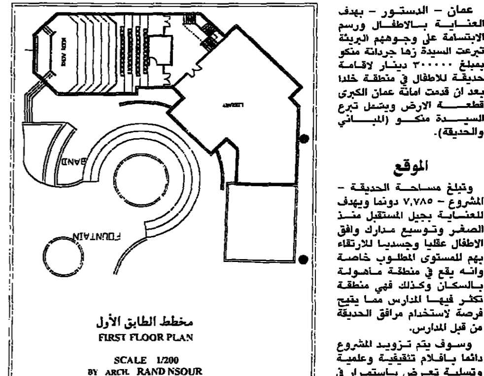
مخطط الطابق الأول GROUND FLOOR PLAN SCALE 1:200 BY ARCH. RAND NSOUR
